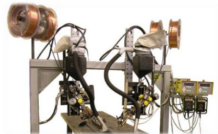
Arco Sumergido
